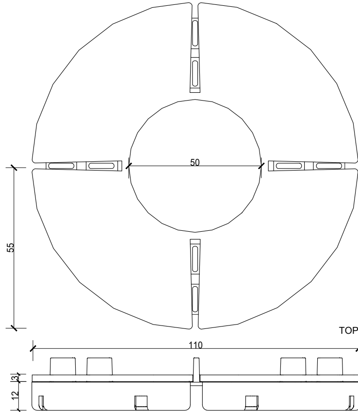
ELEVATION
